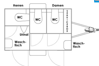
Raumeinteilung bei 3m Länge
