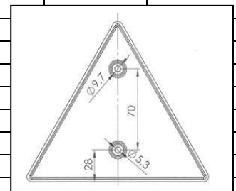
Zeichnung Dreieckrückstrahler
