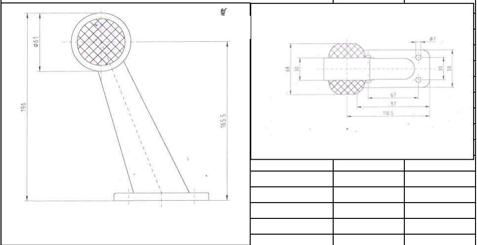
Umrissleuchte links mit Gummihals und Rückleuchte
