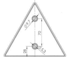
Zeichnung Dreieckrückstrahler
