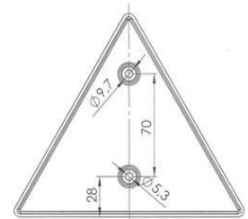
Zeichnung Dreieckrückstrahler
