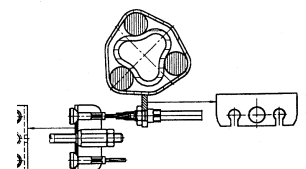
Schnellmontagebowdenzug
