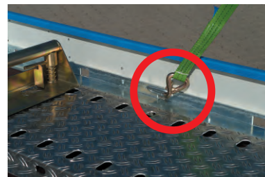
Optimale Verzerrung bei jeder Fahrzeuglänge durch TOPZURR® 22 Zubehör: Verstellkeil auf Aluminium-Arretierblech.
